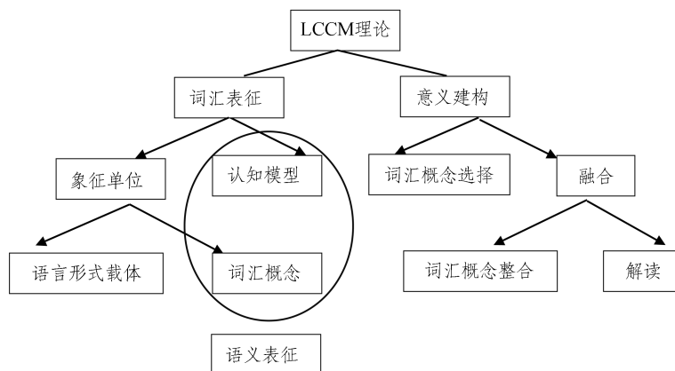
图1 词汇概念与认知模型理论框架
